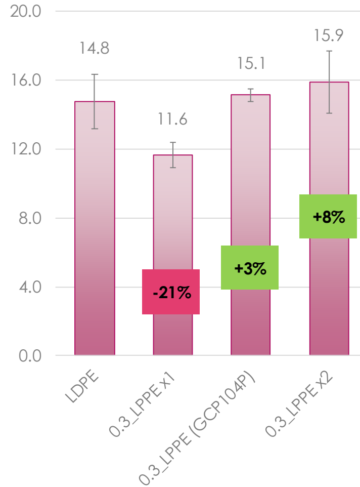
Tensile Strength (MPa)
